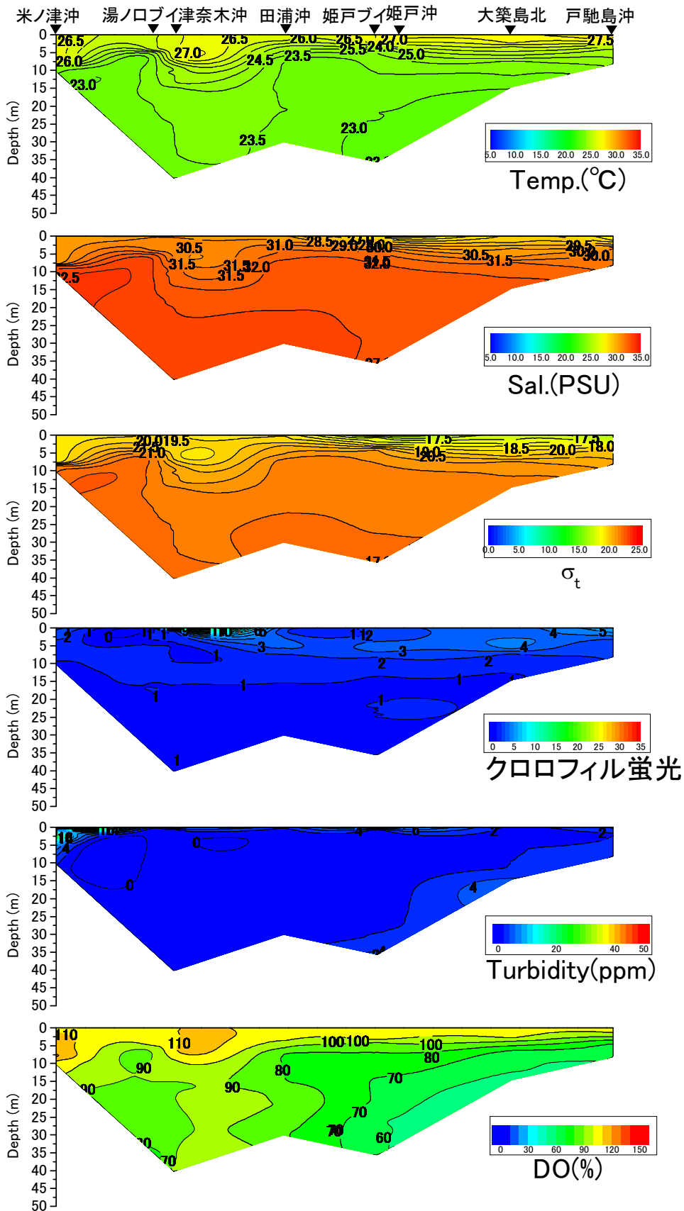
戸馳島沖から米ノ津沖の水温(°C)、塩分、密度( \sigma_t )、クロロフィル蛍光強度、濁度、溶存酸素飽和度(DO%)の鉛直面図(東町漁業協同組合の調査による) (2014年7月31日)
